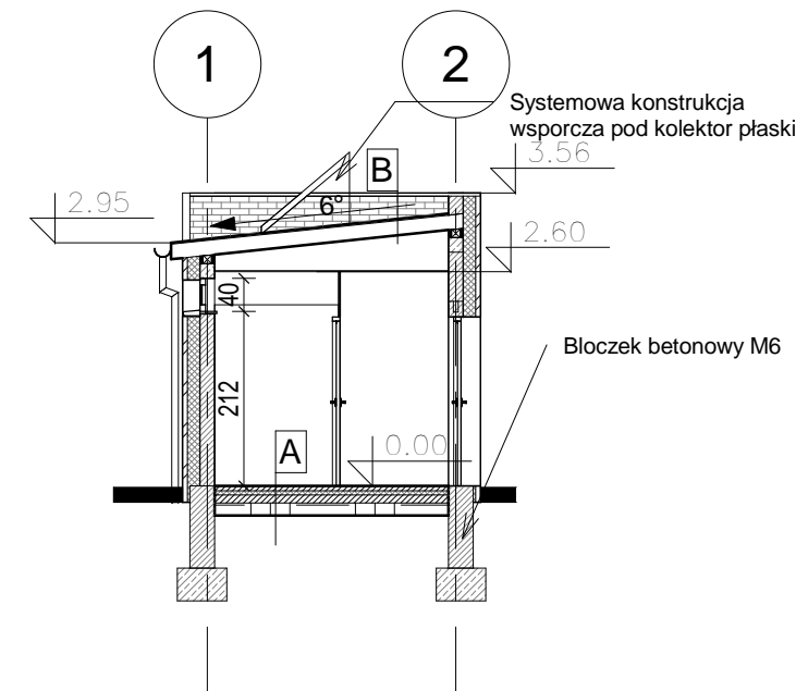
A Przekrój A-A 1 : 100
