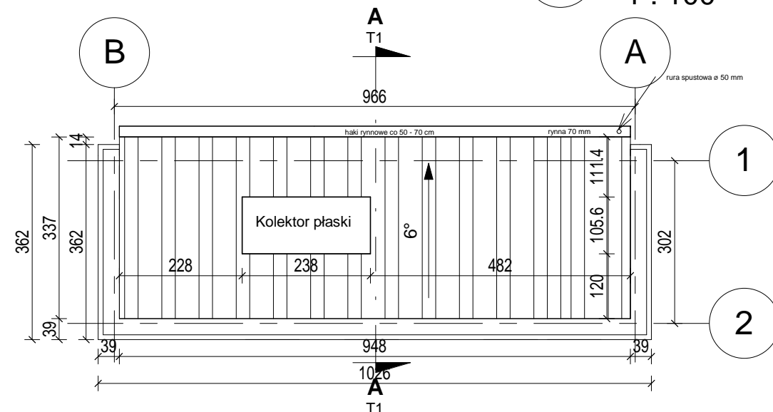
2 Rzut dachu. 1 : 100
