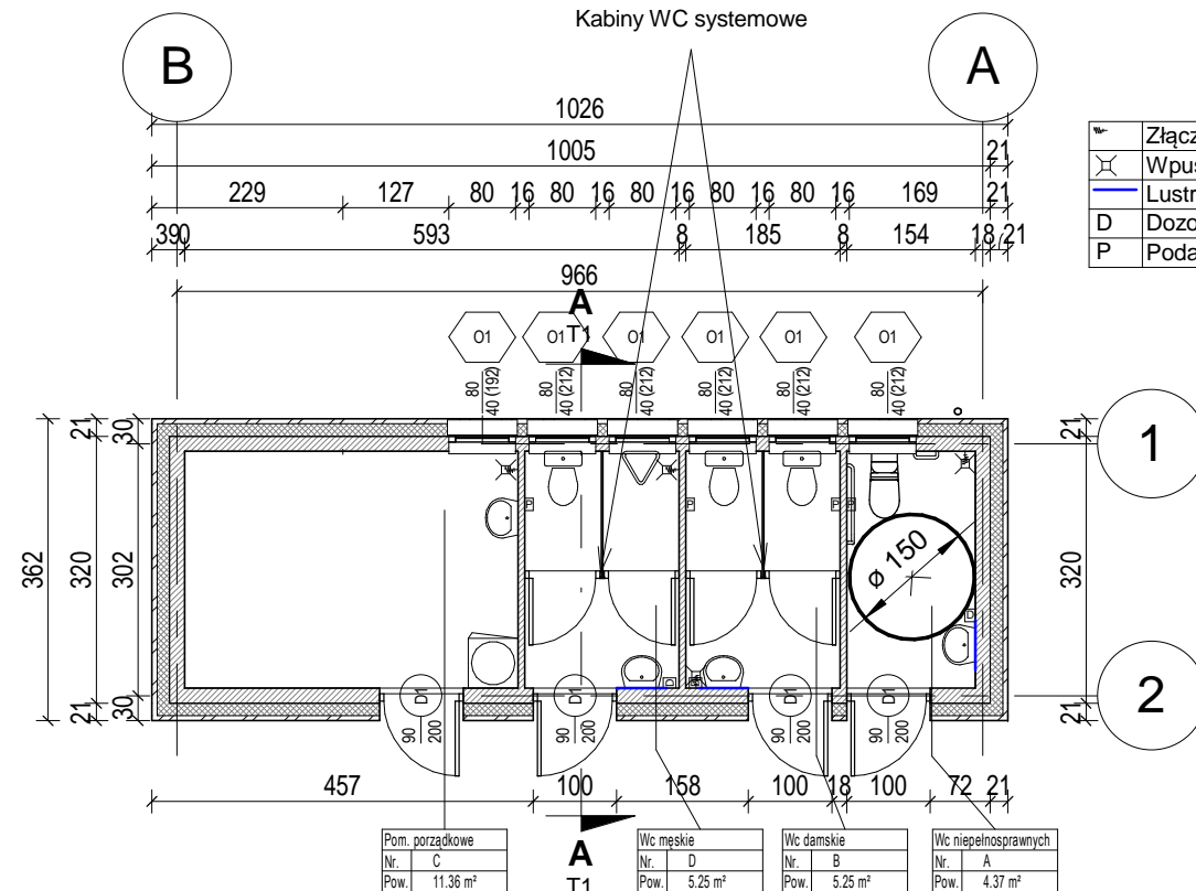
1 Rzut parteru 1 : 100
